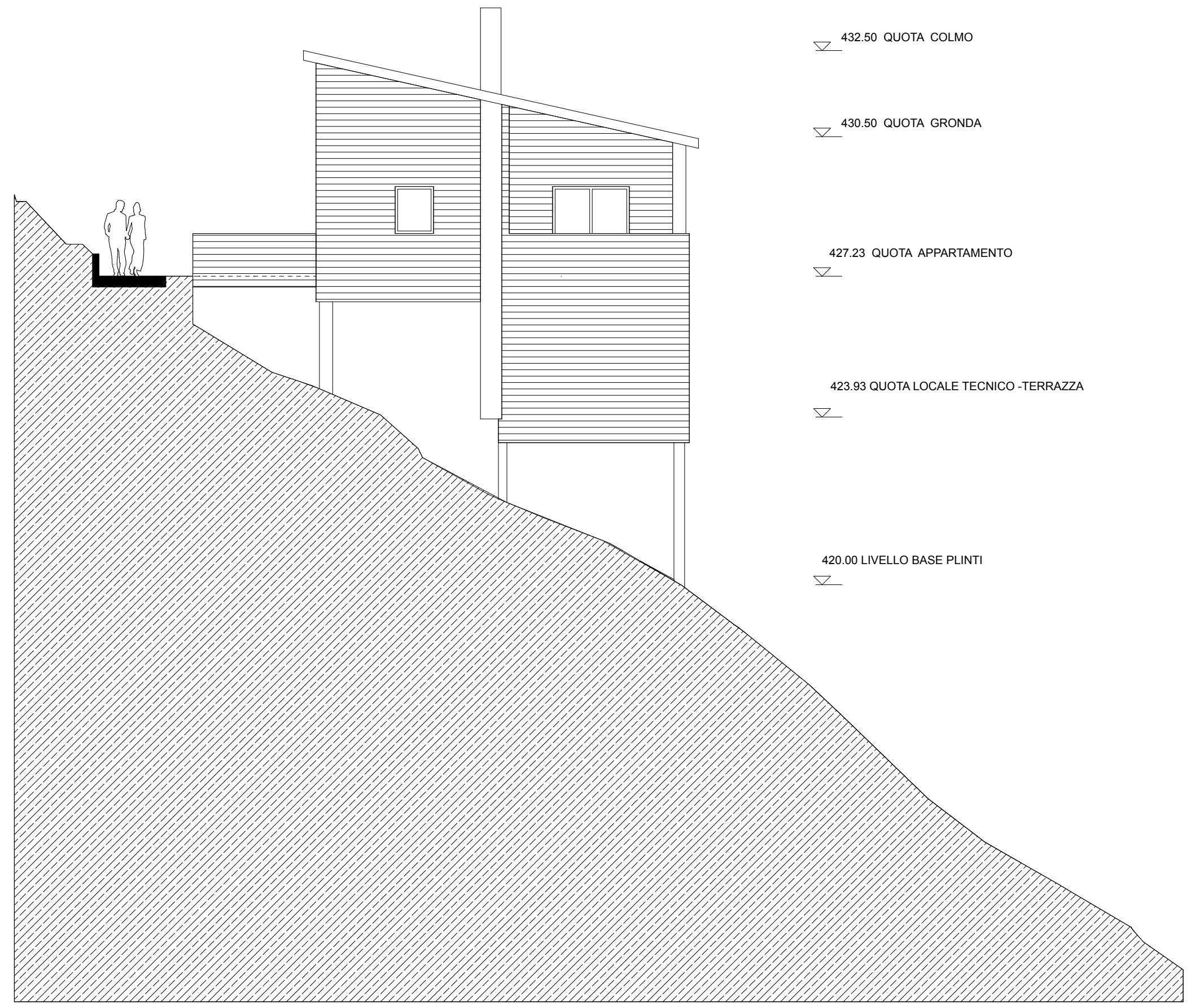
FACCIATA SUD-OVEST
