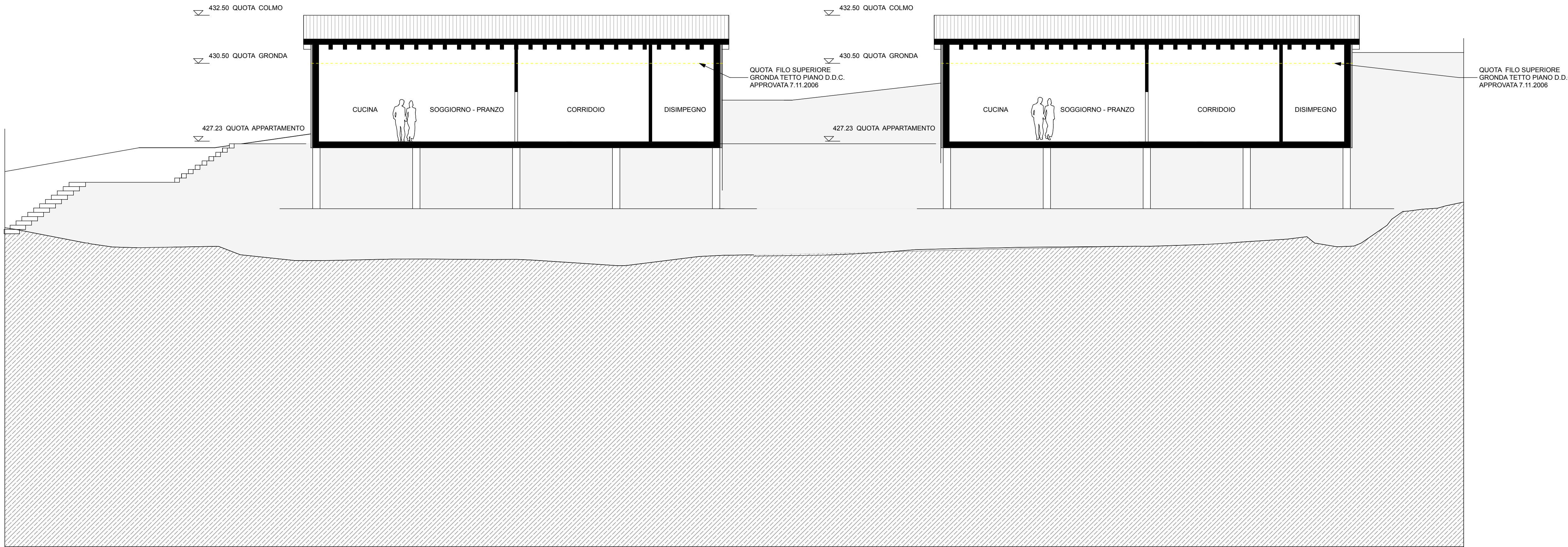
SEZIONE 3A-3B
