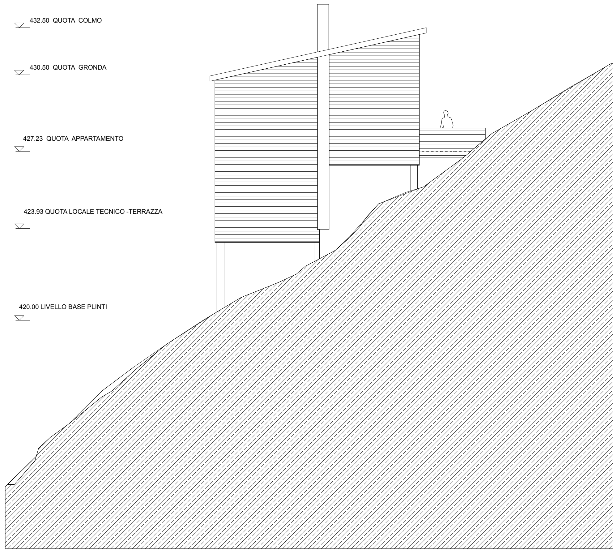
FACCIATA NORD-EST
